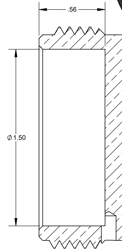
SECTION A-A
