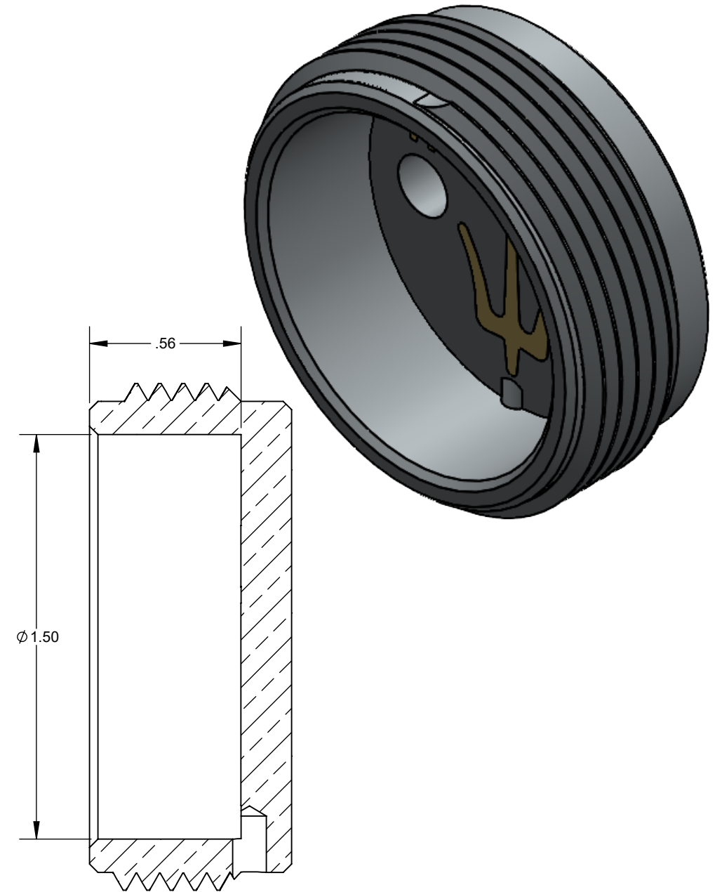
SECTION A-A
