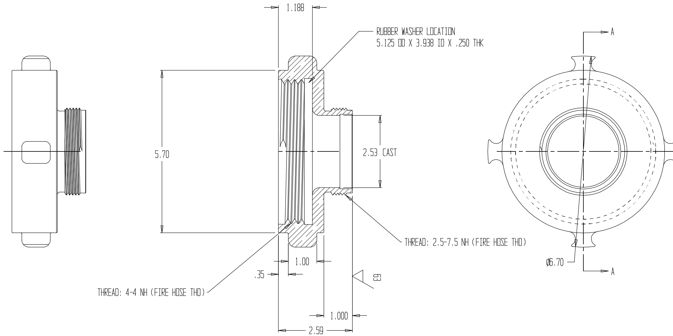
SECTION A-A
